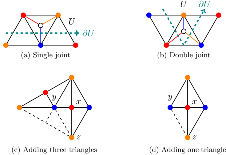
FIGURE 16. Lemma 5.4.
